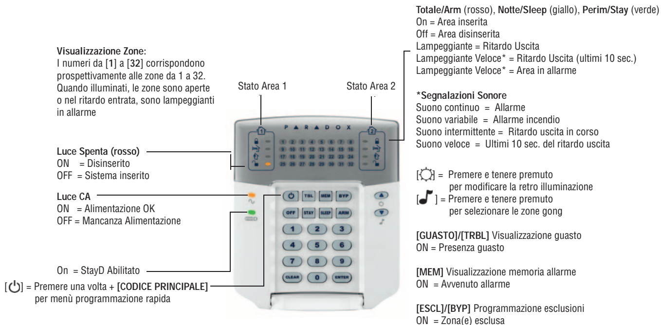
Figura 2 : K32+ (Modulo Tastiera a 32 zone)
